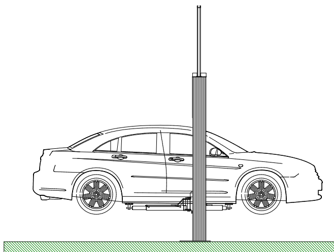
Bild. A) Die Hubsäule muss sich zwischen Lenkrad und den Scharnieren der Autotür befinden
