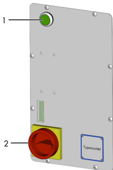
Figura 4: Unidad de mando con conmutador inversor
