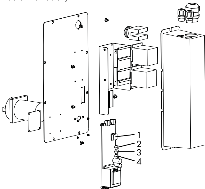
Figura 8: Versión con parada CE 1 Emisor de señal de advertencia 2 R3 Parada CE 3 R1 Arriba apag 4 R2 Abajo apag
