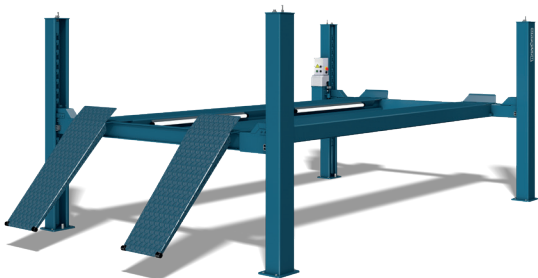
COMBI LIFT estándar con plataformas lisas
